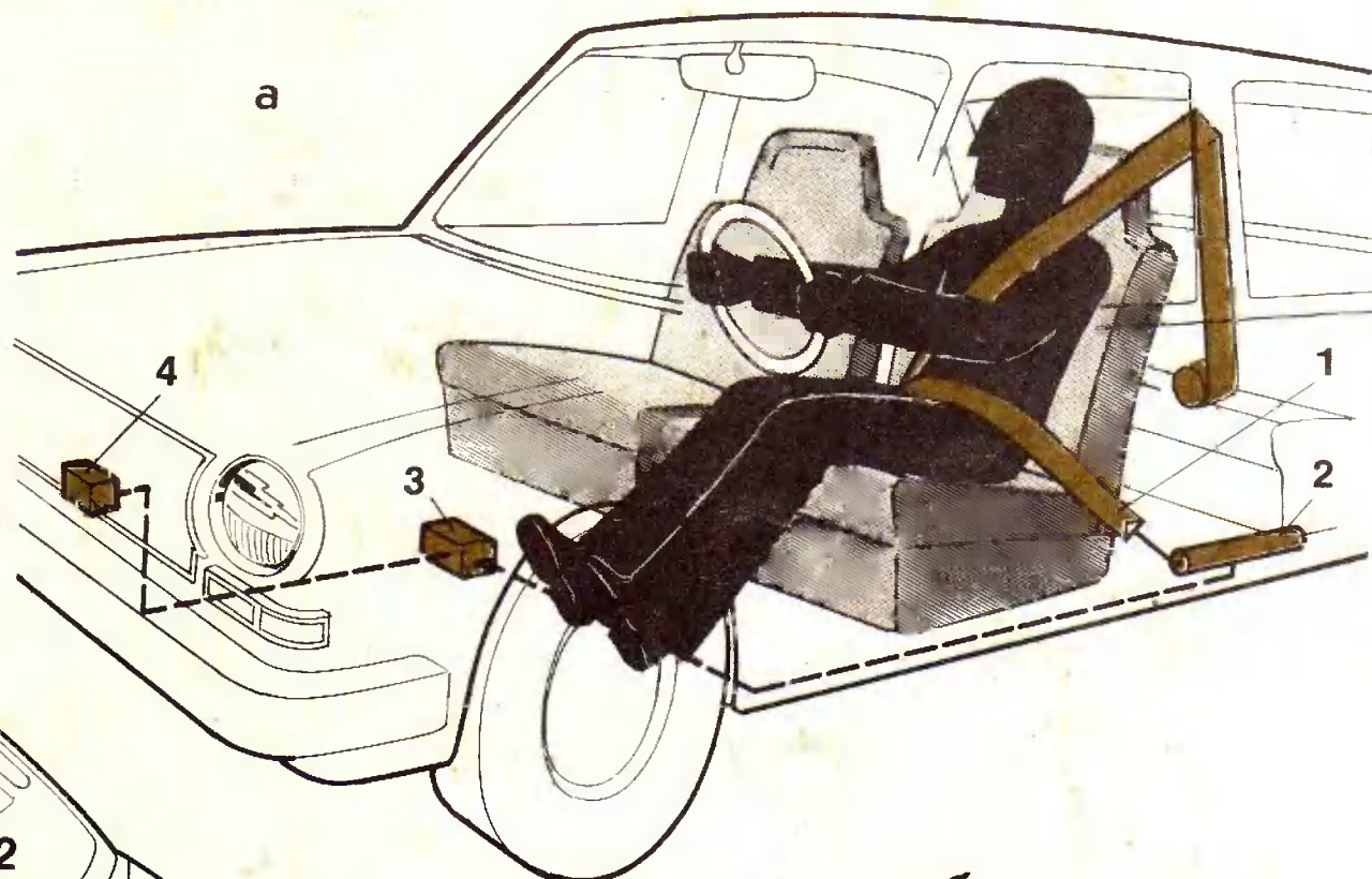
Рис. 1. Система «Даймлер-Бенц» с надувной подушкой и подтягиванием ремней: 1 — подушка; 2 — контрольная лампа; 3 — пиропатрон; 4 — датчик ускорения; 5 — блок управления; 6 — ремень безопасности; 7 — натяжное устройство; 8 — травмобезопасная накладка; 9 — генератор газа; 10 — деформируемый элемент; а — общая схема; б — размещение элементов безопасности в рулевом колесе.
