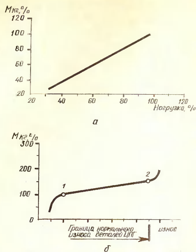
Рис. 1. Зависимость количества газов, прорывающихся в картер M , кг(%): а) от нагрузки; б) от износа деталей цилиндрико-поршневой группы (ЦПГ). Точки: 1 — после обкатки двигателя; 2 — в конце ресурса деталей ЦПГ.
