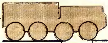
8 МАЗ—535 [СССР, 1—1—1—1].
